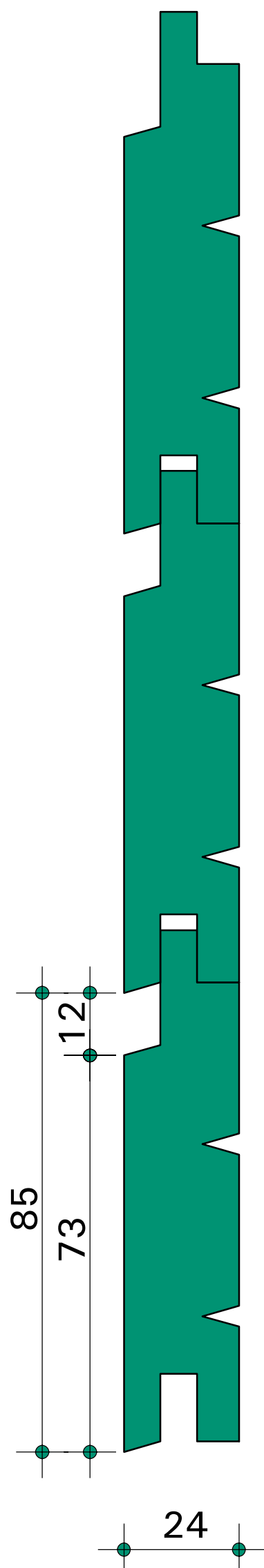
BARDAGE HORIZONTAL Profil Elégie à joint ouvert
