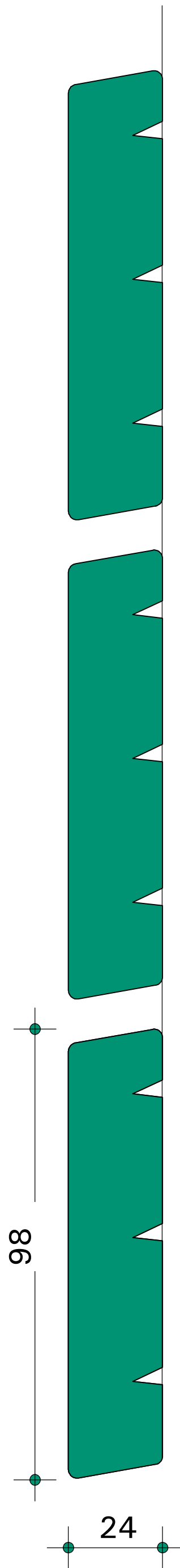
BARDAGE HORIZONTAL Profil Rhomboïde Ajouré Parallélogramme
