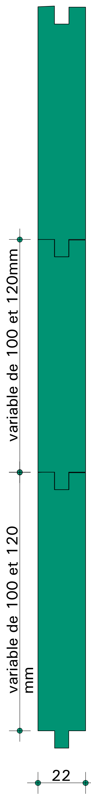
BARDAGE VERTICAL Profil rainé-crête sans chanfrein
